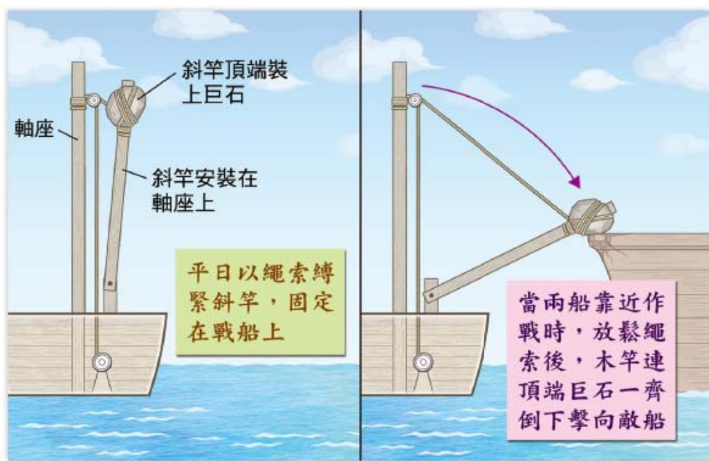
❖ 資料 3 拍竿攻擊原理示意圖
